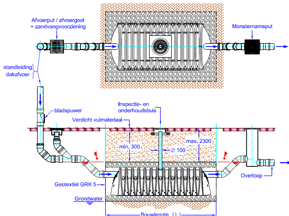
(figuur 1 : Particulier infiltratie voorziening)
