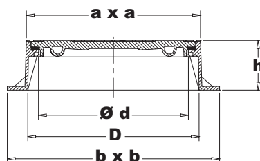
type N 352 NG-R Centerfix Waaiermotief 100 - 175 mm
