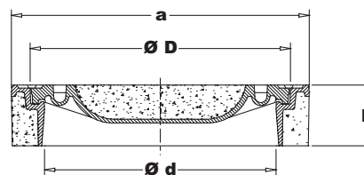
type 7413.70 (B2741370)
