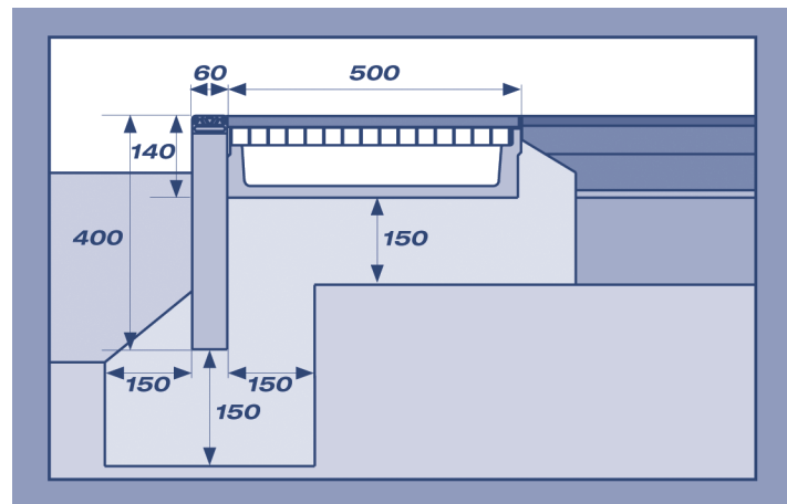
Inbouwvoorbeeld
